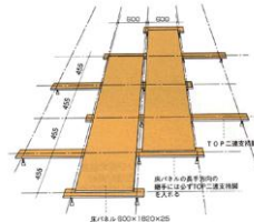
二連支持脚互組工法
