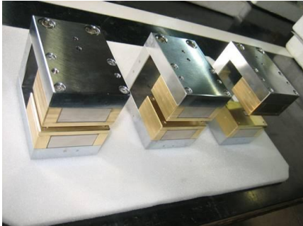
磁場配向用磁気回路（垂直方向磁場）
