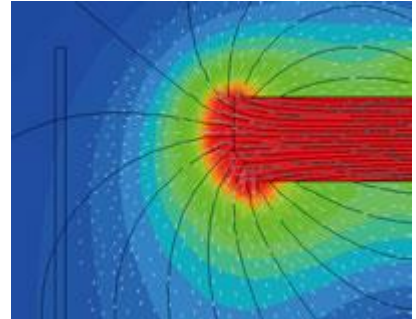
磁場計測
